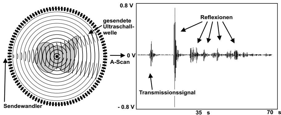
Abb. 1. Funktionsweise eines Ultraschall-Computertomographen, dargestellt in 2D. Ein Wandler sendet einen Puls, alle anderen empfangen die in dem Objekt gestreuten Signale. In dem gezeigten A-Scan sind sowohl das Transmissionssignal als auch Reflexionen an verschiedenen Streuern zu sehen.
